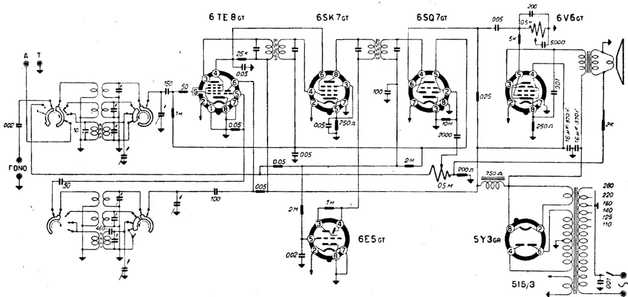
MINERVA RADIO - Mod. 515/3 ADDA - Onde medie e due corte. Media frequenza a 468 kc. Altoparlante da 21 cm. Resa di uscita 3,5 watt. Consumo 55 watt.
